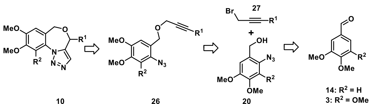
Схема 10. Ретросинтетическая схема синтеза соединений 10 .
