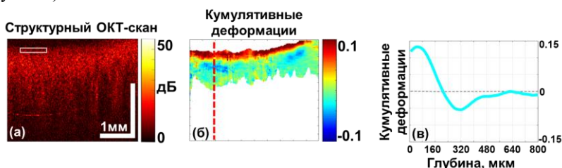
Рисунок 7 — Пример визуализации кумулятивных деформаций осмотической природы, вызванных воздействием на образец хрящевой ткани просветляющего агента «Омнипак» в течение 600 секунд: (а) структурное ОКТ изображение, (б) карта кумулятивной деформации, (в) профиль кумулятивной деформации в глубину вдоль пунктирной линии на (б)
