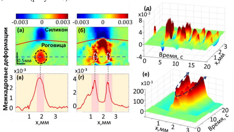
Рисунок 6 — Визуализация межкадровых и накопленных (кумулятивных) деформаций на основе развитой фазочувствительной ОКТ-технологии в роговице глаза кролика при облучении ее импульсно-периодическим излучением инфракрасного лазера с длиной волны 1.5 мкм. Панель (а) - двумерное распределение межкадровой деформации в роговице по глубине в начале нагревающего импульса, когда скорость деформации первоначально максимальна на оси пучка. Панель (б) - межкадровая деформация, зарегистрированная на \sim 2 с позже, когда скорость деформации имеет уже два максимума на склоне температурного распределения. Графики (в) и (г) показывают соответствующие горизонтальные профили деформации вдоль пунктирных линий, показанных на панелях (а) и (б). Из профилей хорошо видно, что формы распределения деформации первоначально имеют один центральный максимум, а затем формируются даже более интенсивные расщепленные максимумы на более поздней стадии нагрева. Панель (д) представляет временную эволюцию межкадровых деформаций при импульсно-периодическом нагреве роговицы. Отчетливо виден постепенный переход от изначально одного центрального максимума к расщепленным максимумам на склонах греющего пучка. Панель (е) соответствуют панели (д), но показывает уже эволюцию накопленных (кумулятивных) деформаций, также демонстрирующих расщепление первоначально единственного максимума и формирование двух боковых максимумов, значительно превышающих по амплитуде центральный
