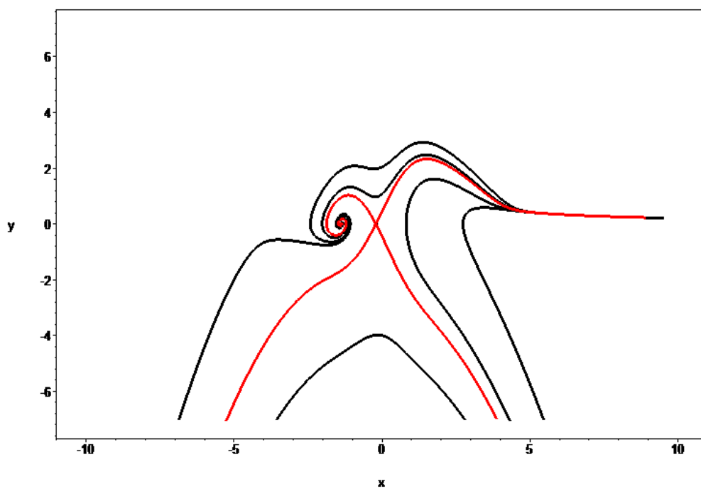
Рис. 3.5.14. Квадратичная добавка, \tau > 0 , неустойчивый фокус и седло.
