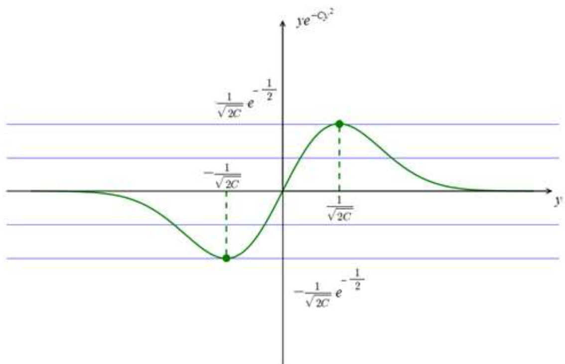
Рис. 3.5.1. Вид решений системы (3.5.10).
