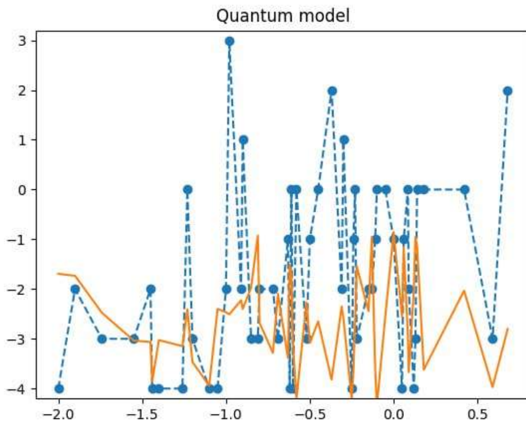
Рис. 2.3.15. Данные эксперимента (пунктирная линия) и результаты моделирования (сплошная) с параметрами, подобранными методом наименьших квадратов.
